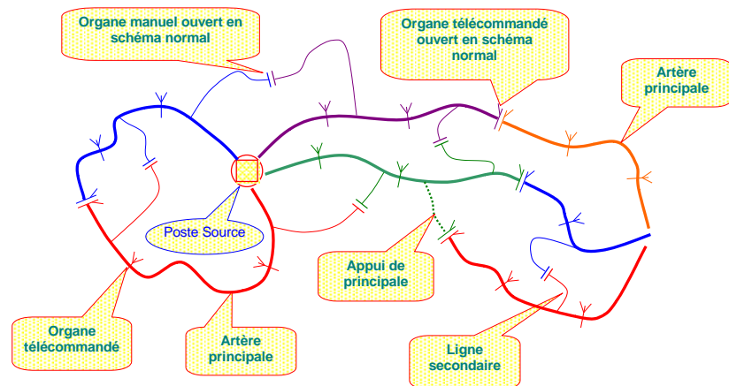
Figure 4 : Détermination des principales avec leur organe télécommandé de bouclage
