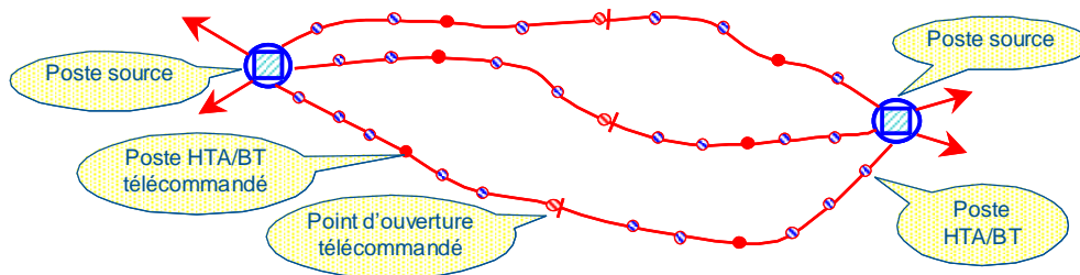
Figure 5 : exemple de structure en coupure d'artère
