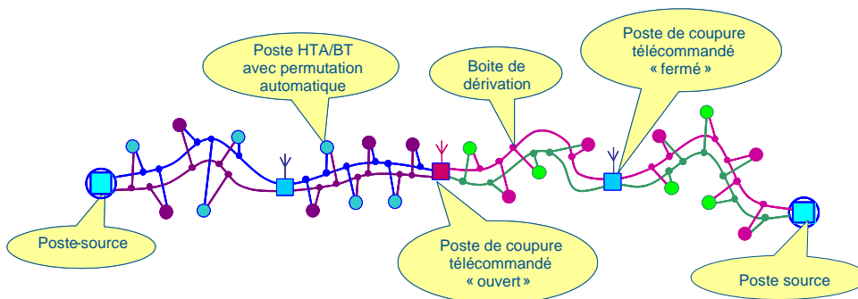
Figure 6 : exemple de structure en double dérivation
