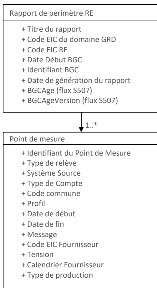
Diagramme de classes UML des flux S507
