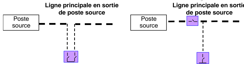
Figure 14 : Interrupteur pour faciliter la réalimentation en cas de mise hors tension du poste source
