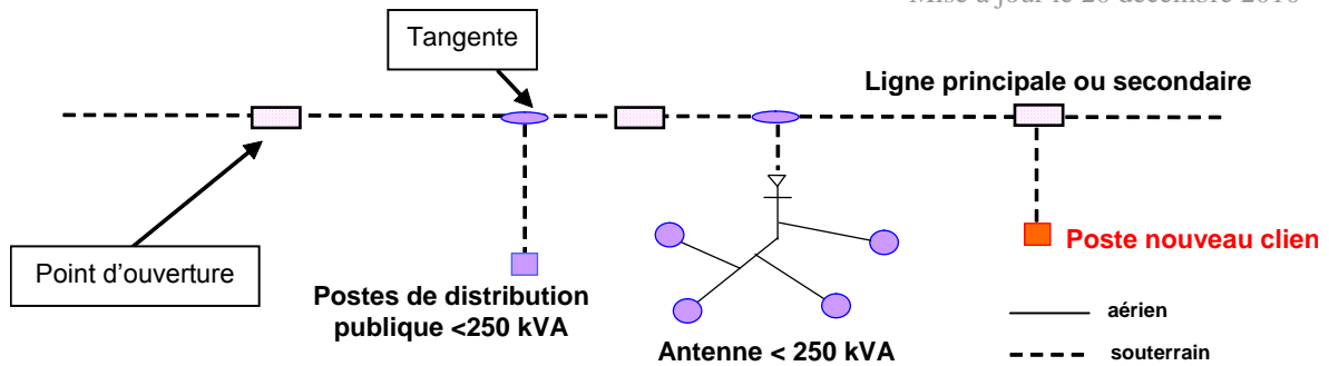
Figure 11 : Illustration de la règle d'une tangente maximum entre deux points d'ouverture
