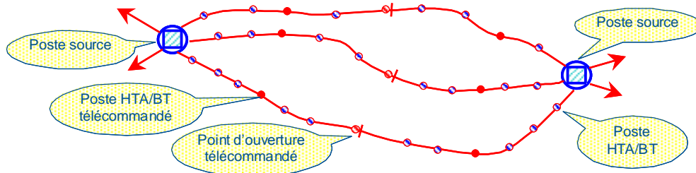
Figure 5 : exemple de structure en coupure d'artère
