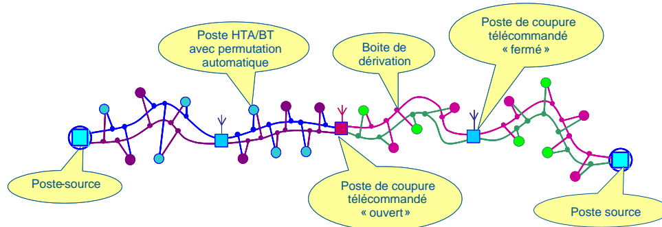
Figure 6 : exemple de structure en double dérivation
