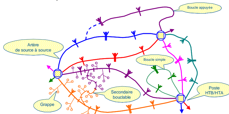
Figure 7 : Structure de réseau rural
