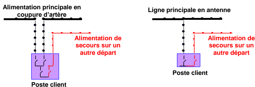
Figure 15 : Schémas d'alimentation pour une alimentation de secours
