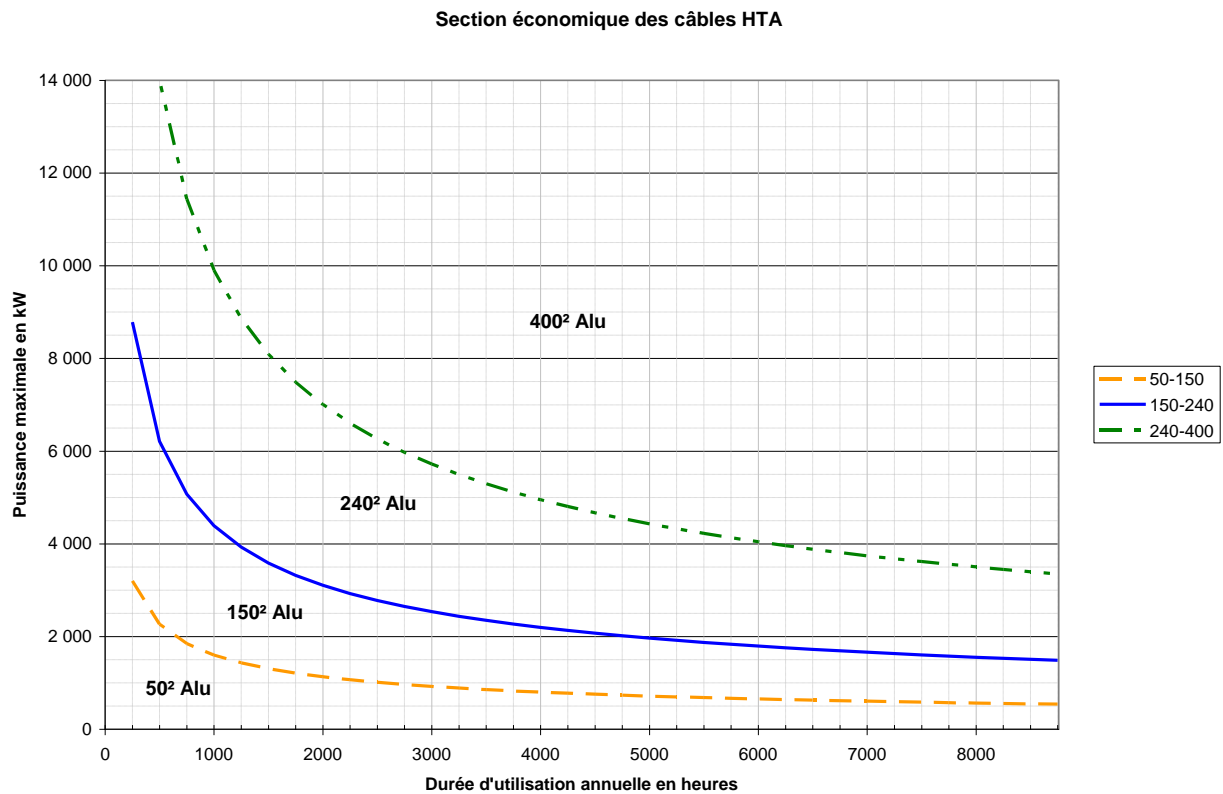
Figure 9 : Abaques des sections économiques de câble (ne prenant pas en compte les intensités admissibles)
