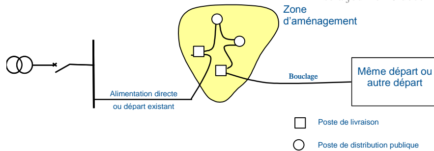
Figure 3 : Exemple de structure de réseau d'alimentation d'une ZAC
