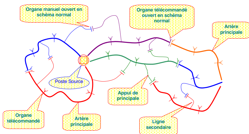
Figure 4 : Détermination des principales avec leur organe télécommandé de bouclage
