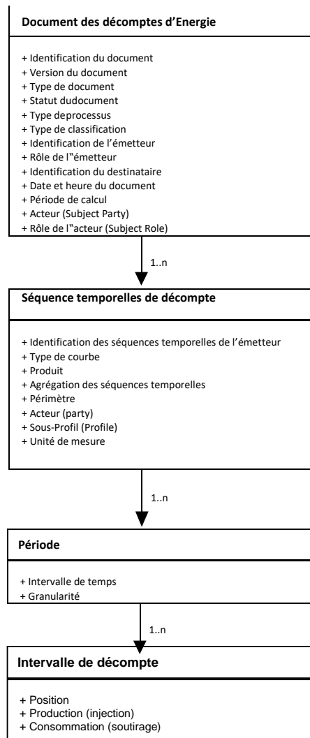
Diagramme de classes UML des flux S503
